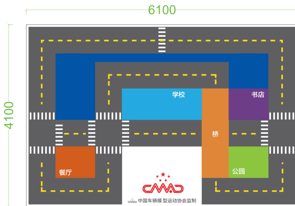
图23 无人驾驶智能车任务赛场地示意图
