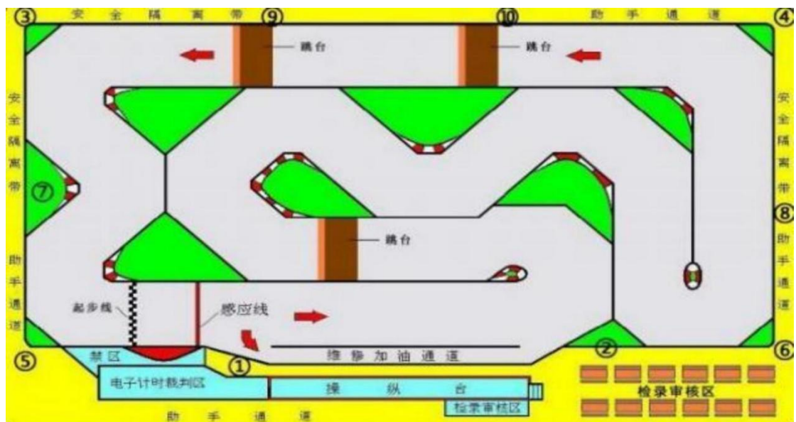
图16 1/10电动平跑车（无跳台）、1/16电动平跑车（无跳台）、1/18电动平跑车（无跳台）、1/18电动越野车竞速赛场地示意图
