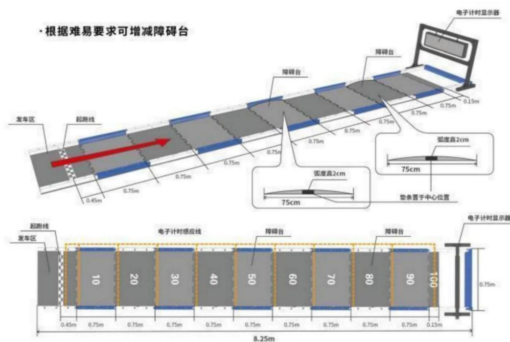
图6 空气动力竞速赛场地示意图
