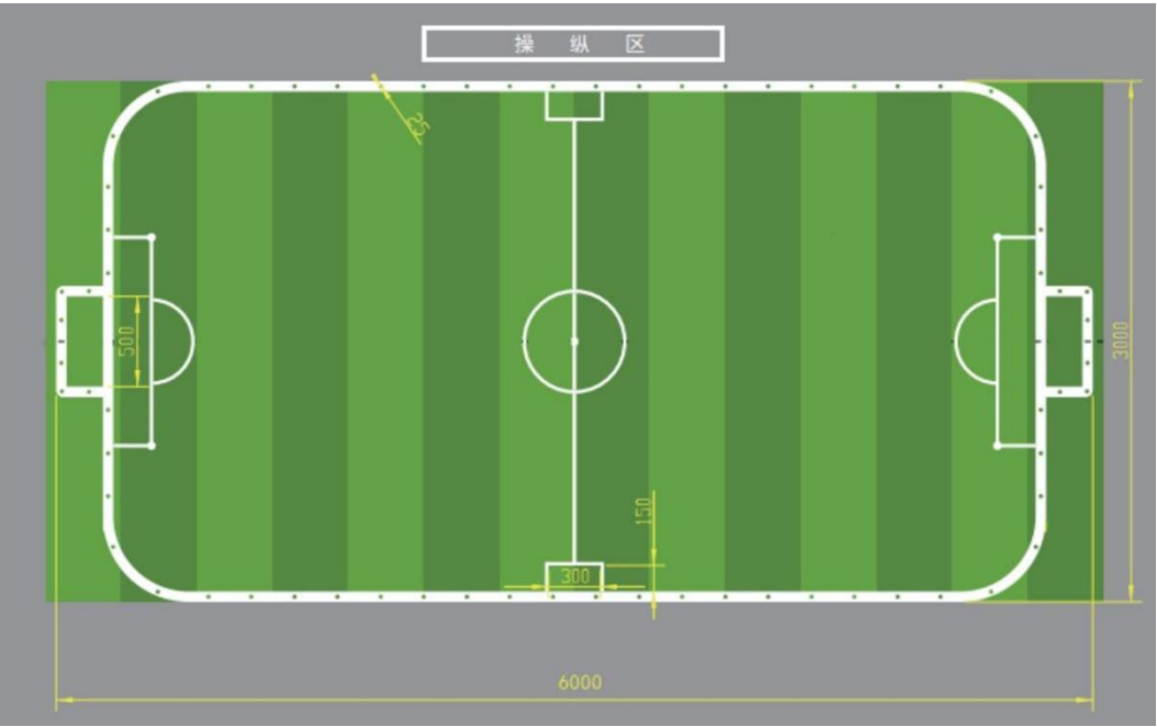
图14 迷你足球赛（团体）场地示意图
