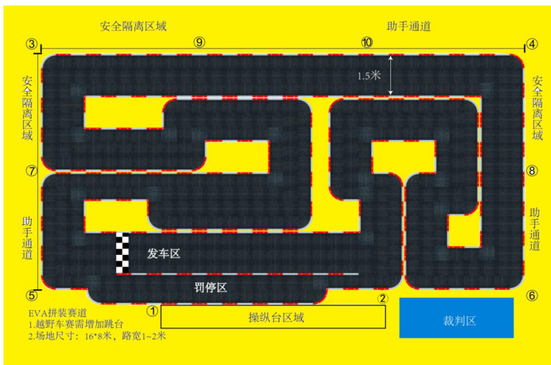
图21 1/18电动方程式、1/18电动公路车、1/22、1/24电动拉力车竞速 场地示意图
