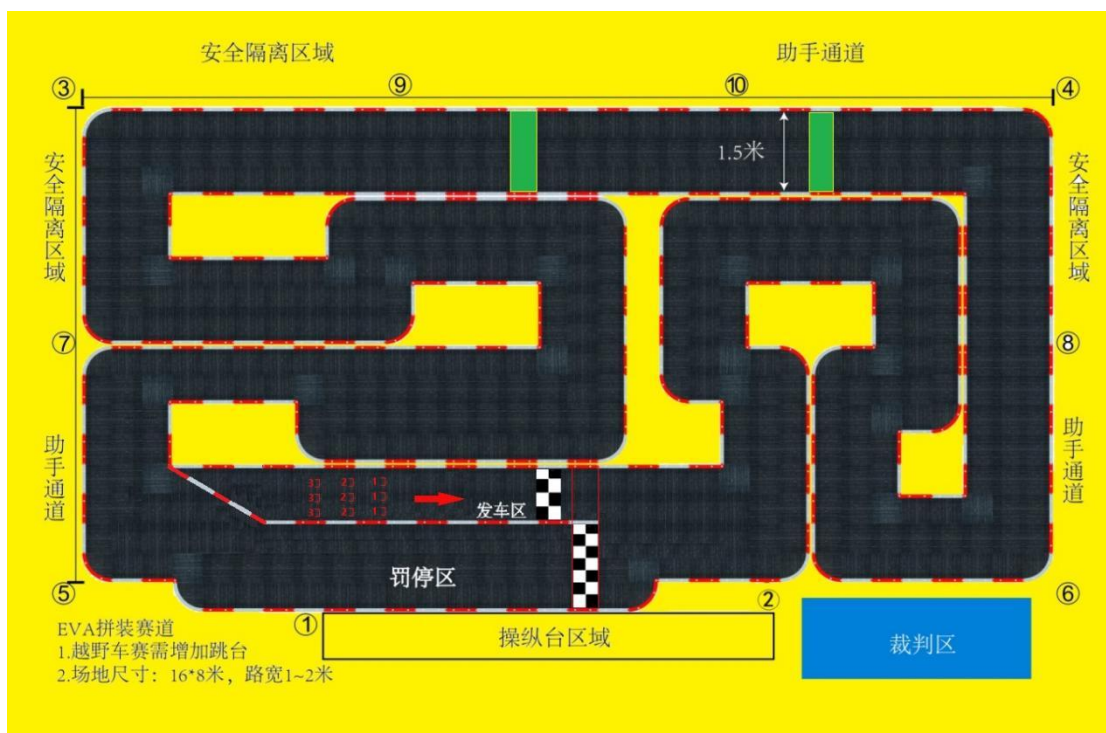
图19 1/24电动拉力车（团体）（无跳台）、1/24电动越野车竞速赛（团体）场地示意图
