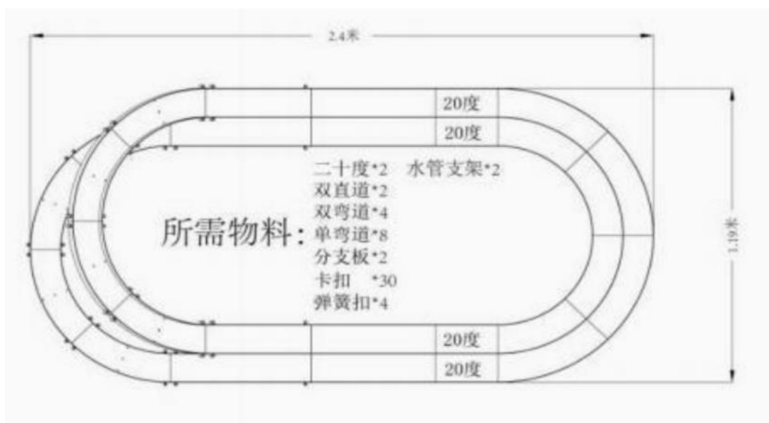
图5 四驱车调试场地示意图
