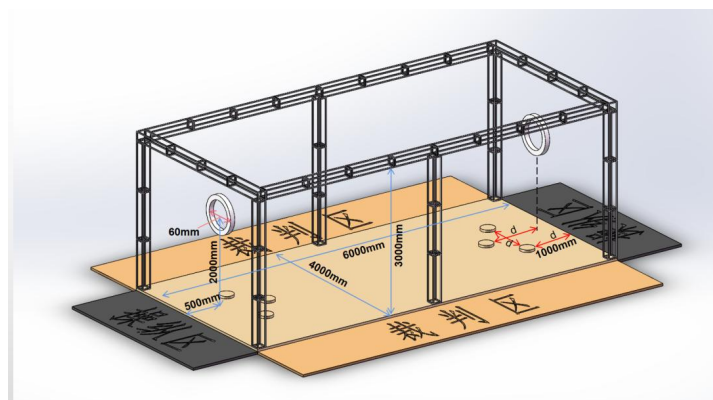
图十九：遥控纸质四轴飞行器空中足球对抗赛场地示意图
