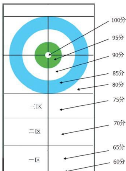
图 5-1 分值示意图
