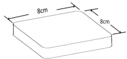
图一 承压垫板
