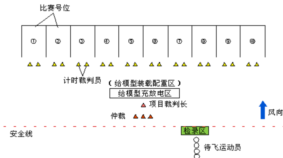
图 1 竞时和弹射项目竞赛场地示意图
