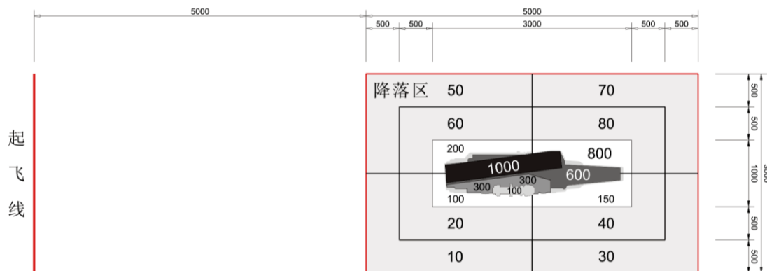
图4 仿真纸飞机航母着舰积分赛场地示意图（单位：毫米）
