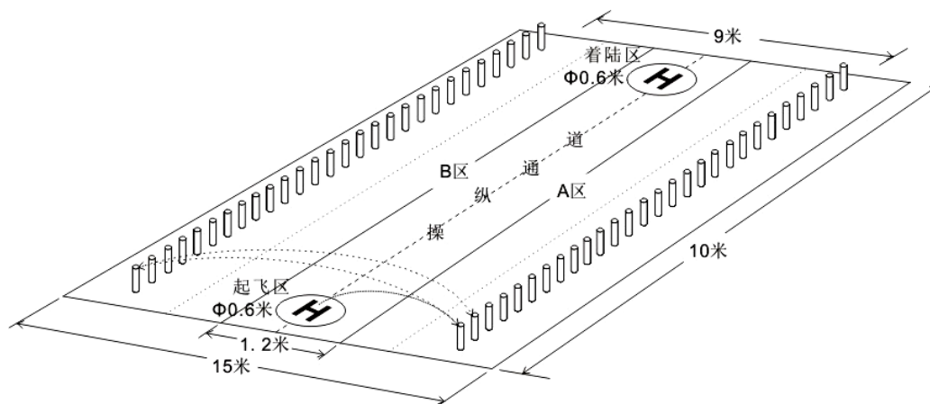
遥控直升机任务飞行场地示意图
