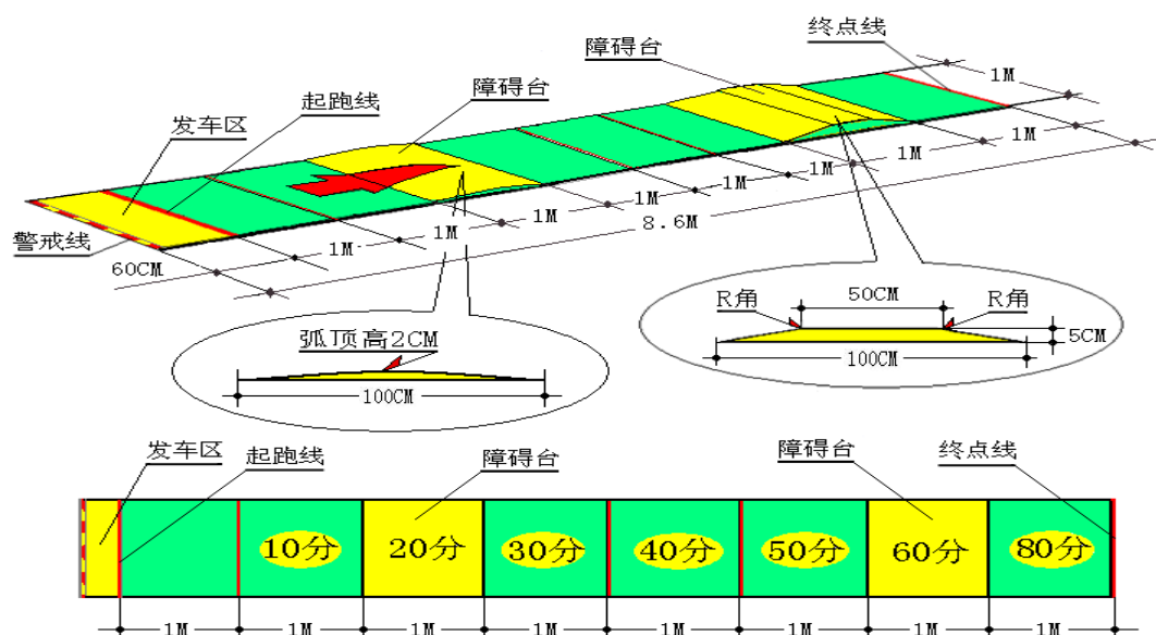
太阳能车竞速赛道示意图
