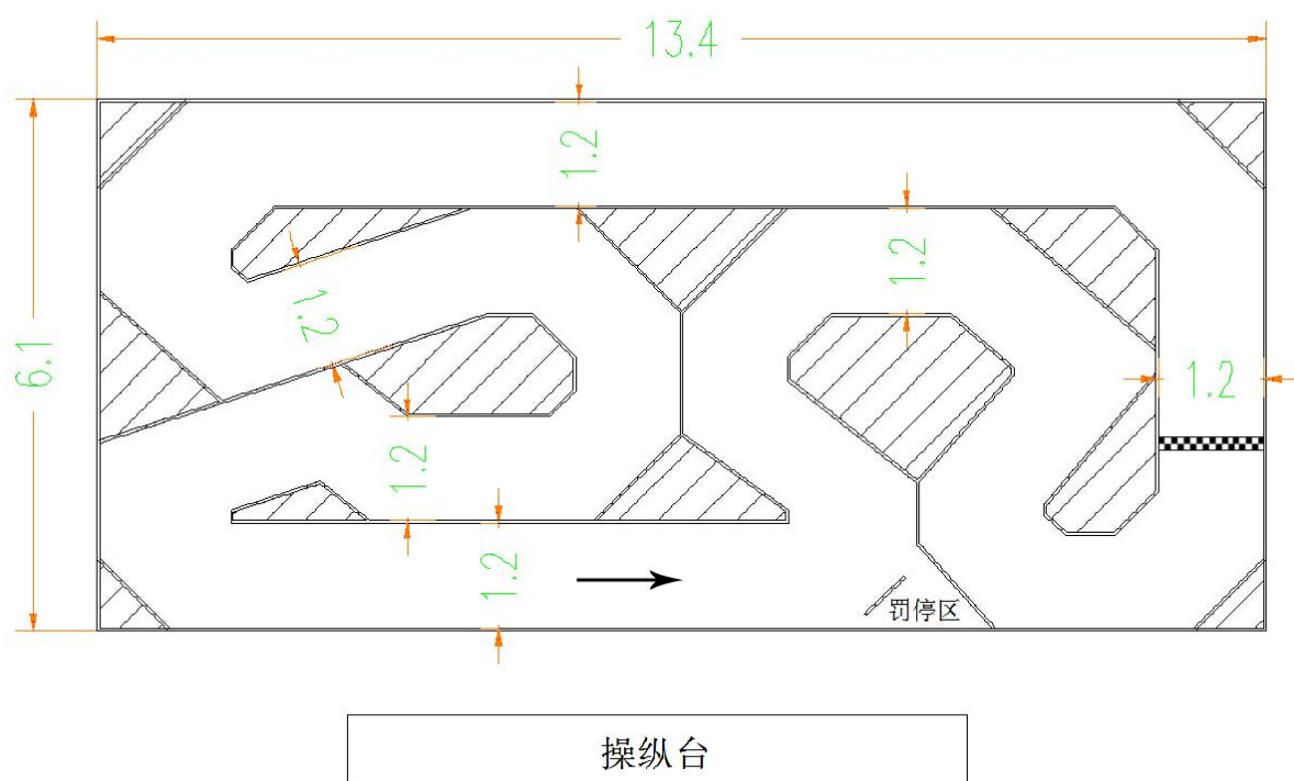
1/18 遥控电动房车竞速赛、1/24 遥控电动拉力车竞速赛竞赛场地图
