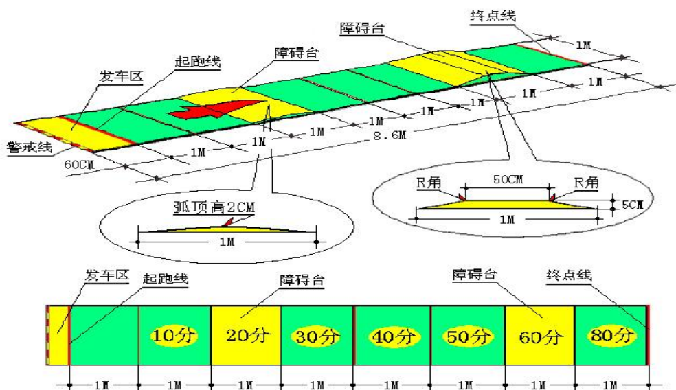
橡筋动力车拼装直线赛道示意图
