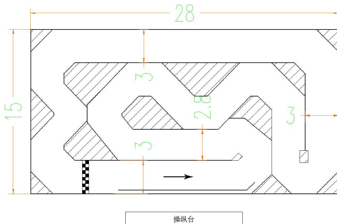
1/14 遥控电动平跑车竞速赛、1/16 遥控电动房车竞速赛、1/16 遥控电动越野车竞速赛竞赛场地图
