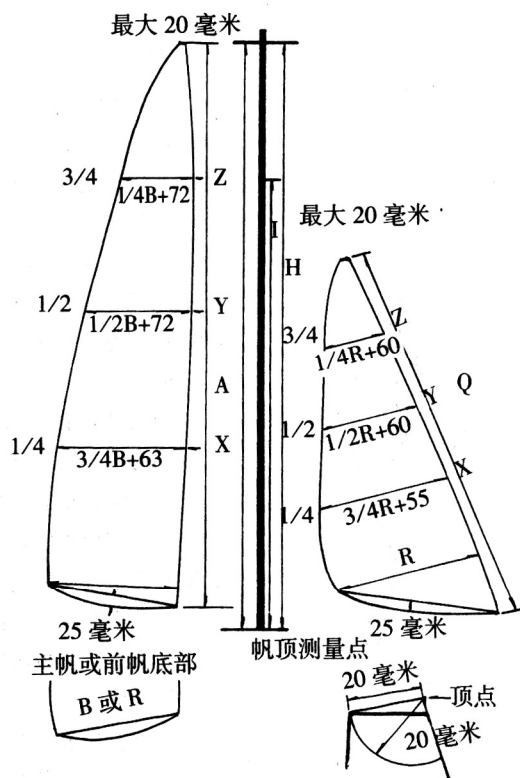
M 级 帆面积测量图
