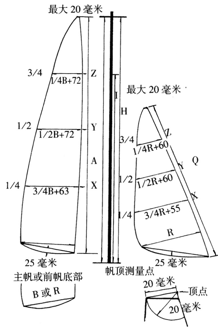
M 级 帆面积测量图
