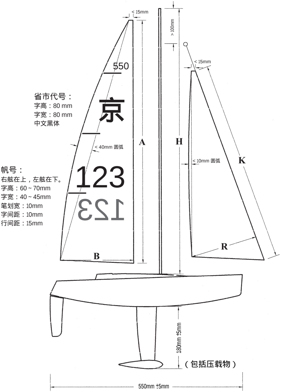
F5 550 级 帆面积测量图
