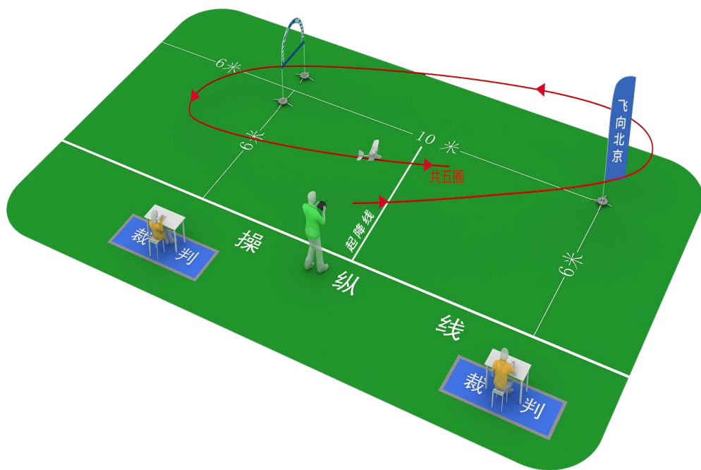
图 14 微型双翼遥控模型飞机趣味飞行场地示意图
