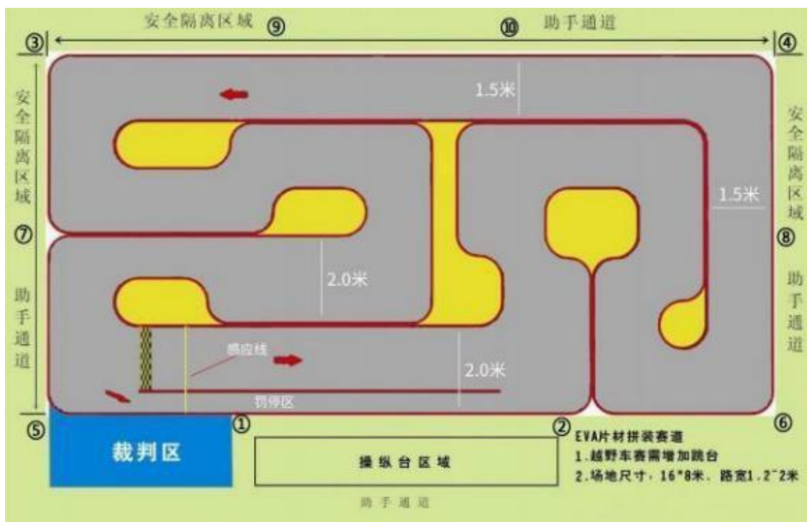
图4 1/24 电动拉力车比赛场地示意图
