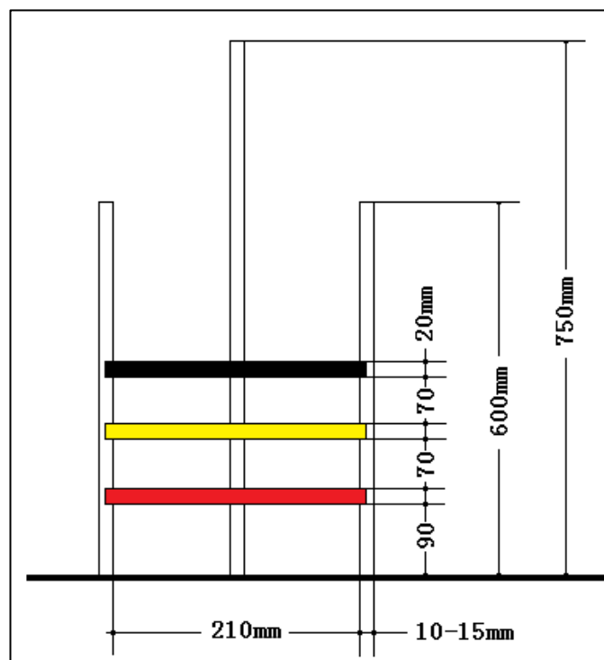
图 7 漂移项目得分区示意图
