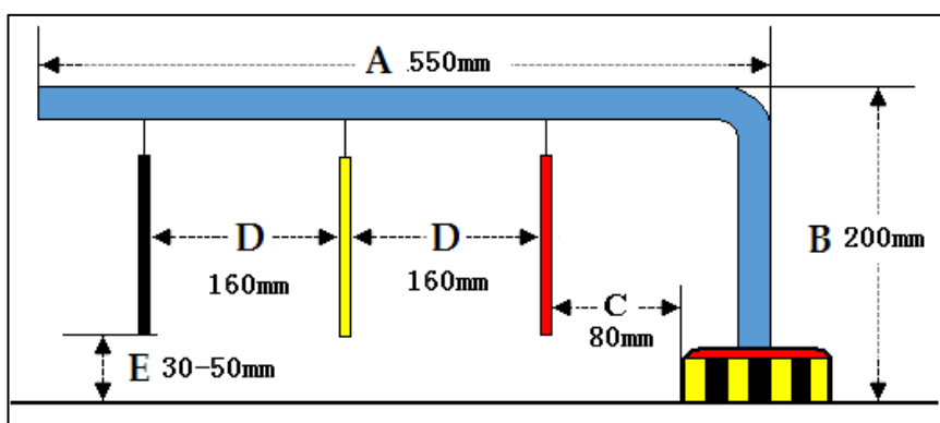
图 6 漂移项目得分杆示意图
