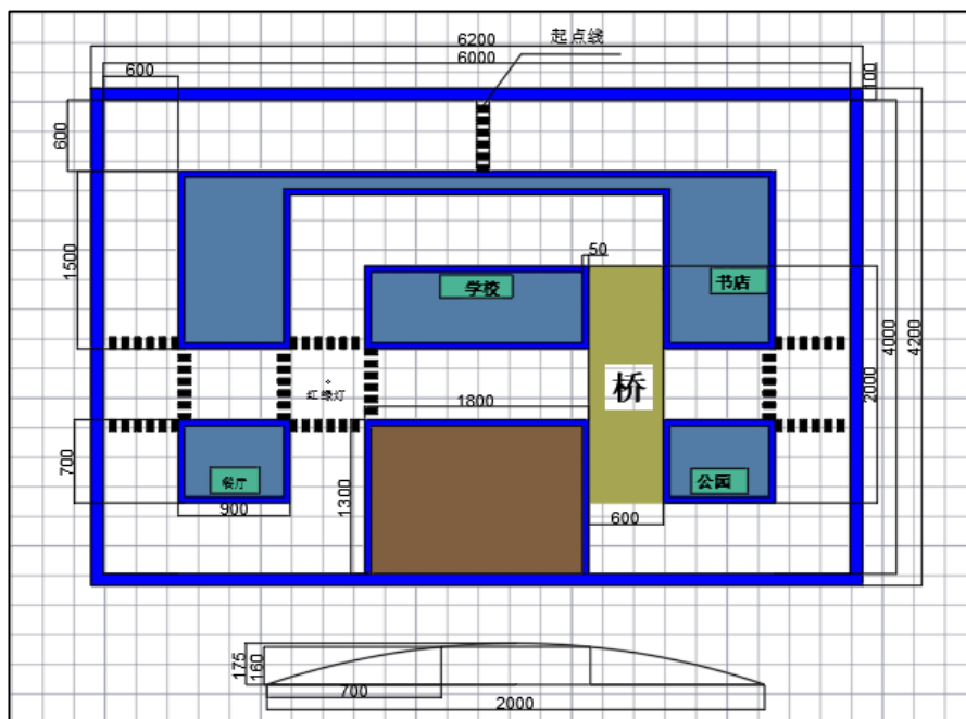
图 10 智能无人驾驶车积分赛场地示意图
