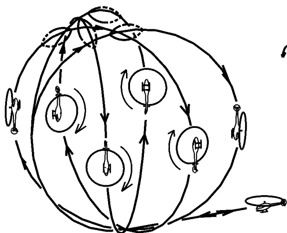
B.5 GALAXY
