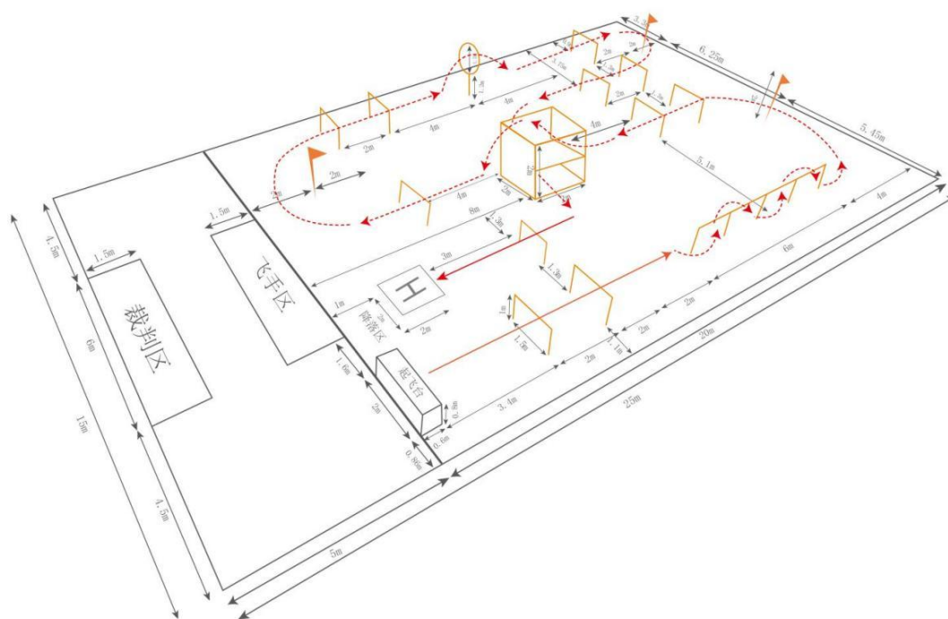
多轴无人机竞速场地示意图
