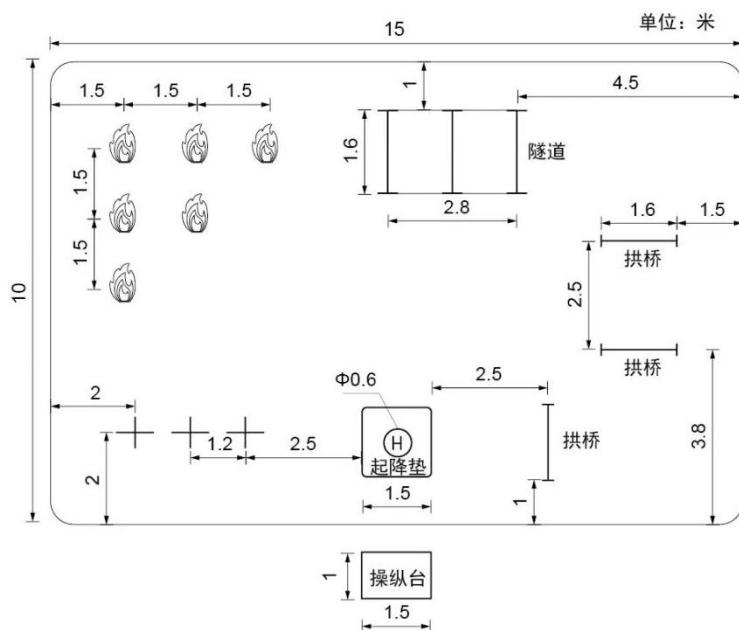
多轴无人机花式飞行场地示意图
